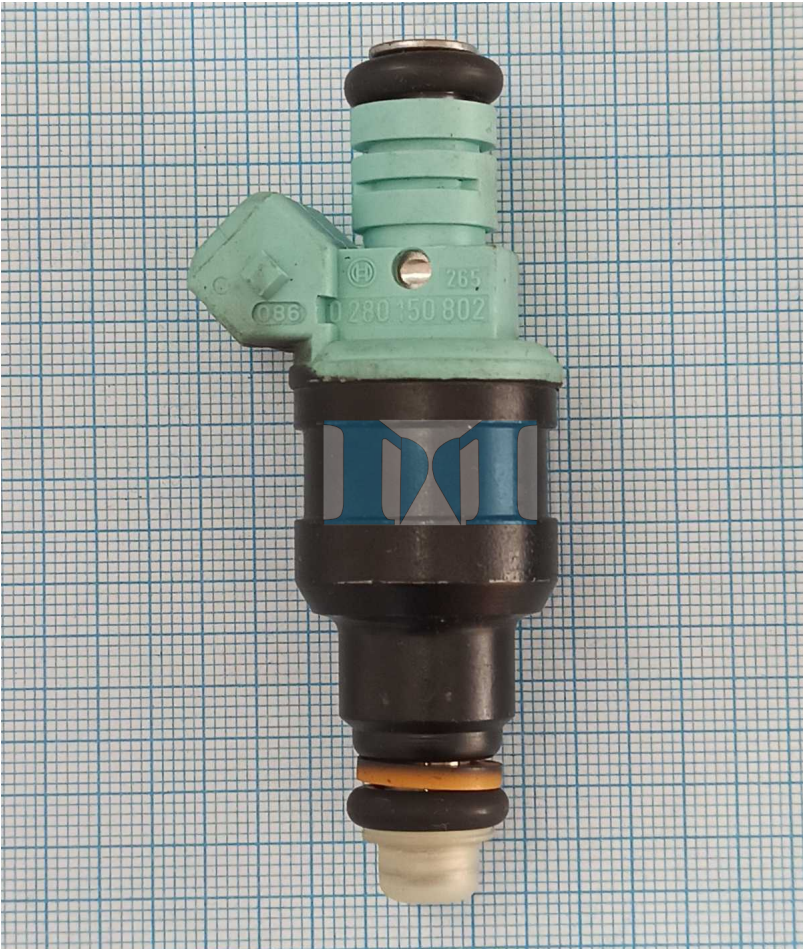
???? ?? ?????????? BOSCH - 0280150802
